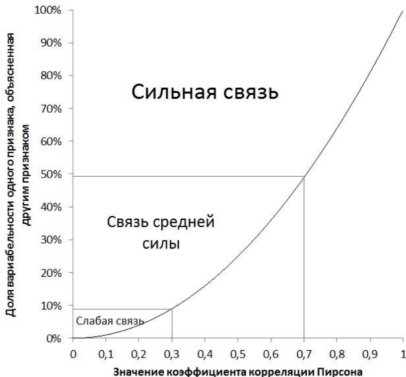
Рис. 2. Зависимость значения коэффициента детерминации от значения коэффициента корреляции.
