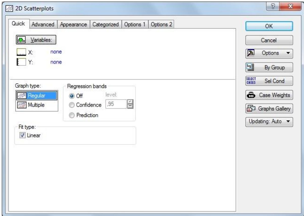
Рис. 3. Окно «2D Scatterplots» программы Statistica 10.
