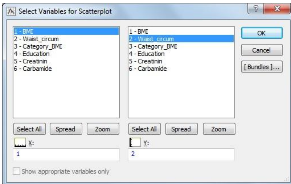
Рис. 4. Окно «Select Variables for Scatterplot» программы Statistica 10.
